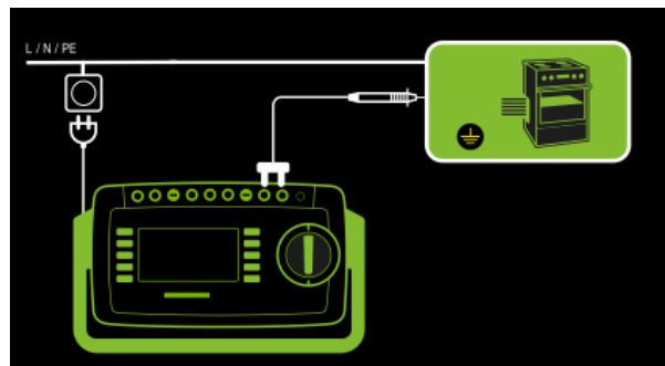
Abb. 48: Prüflinge der Schutzklasse I – Sonderfall fest installierte Prüflinge, Anschlussschaltbild
