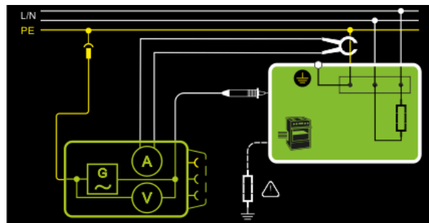
Abb. 49: Messung über Zangenstromsensor an fest installierten Prüflingen, Prinzipschaltbild
