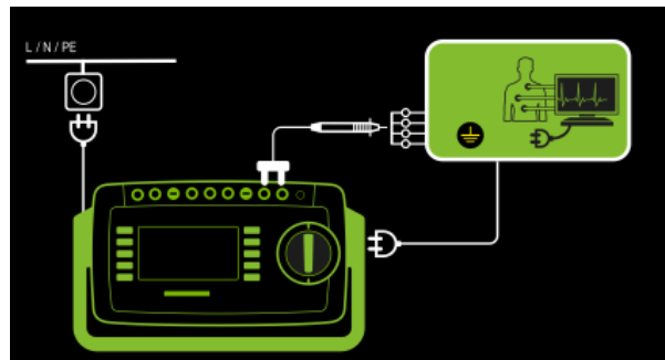
Abb. 124: Direktes Messverfahren, Anschlussschaltbild
