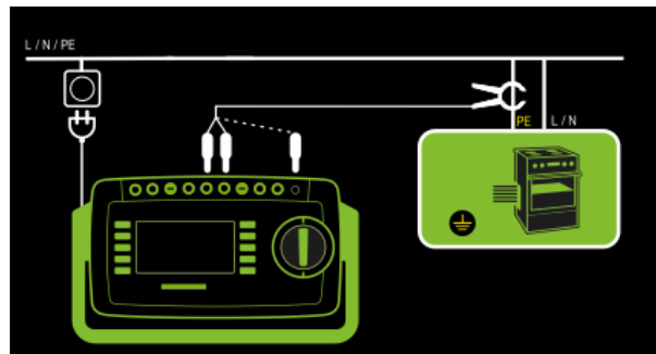
Abb. 92: Messung des Schutzleiterstroms über Zangenstromsensor mit Spannungsausgang bei fest installierten Prüflingen, Anschlussschaltbild (Zangenstromsensor an COM-V)
