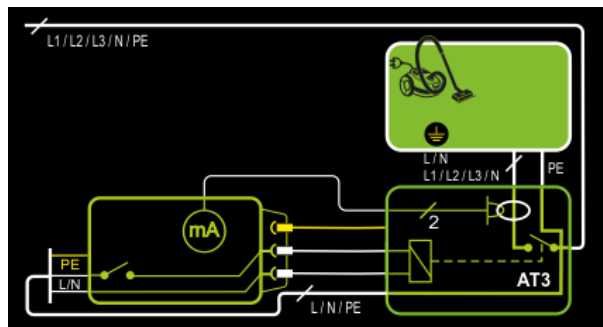
Abb. 89: Anschluss von 3-phasigen Prüflingen, Prinzipschaltbild
