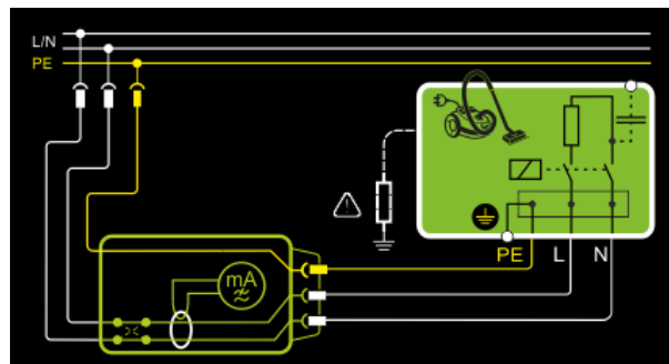
Abb. 85: Differenzstrommessverfahren, Prinzipschaltbild
