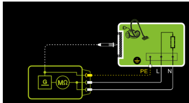
Abb. 70: Prüflinge der Schutzklasse I mit berührbaren elektrischen Teilen, Prinzipschaltbild
