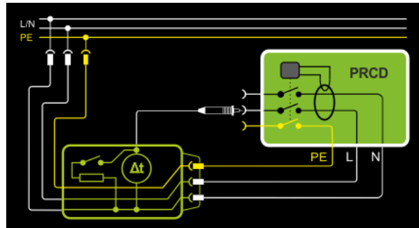
Abb. 137: Messung der Auslösezeit von Fehlerstrom-Schutzeinrichtungen, Prinzipschaltbild
