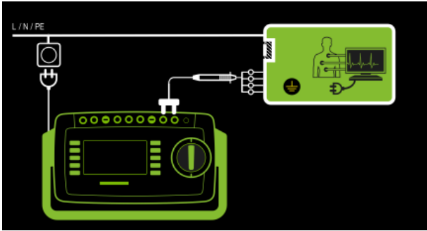
Abb. 121: Direktes Messverfahren, Anschluss Schaltbild
