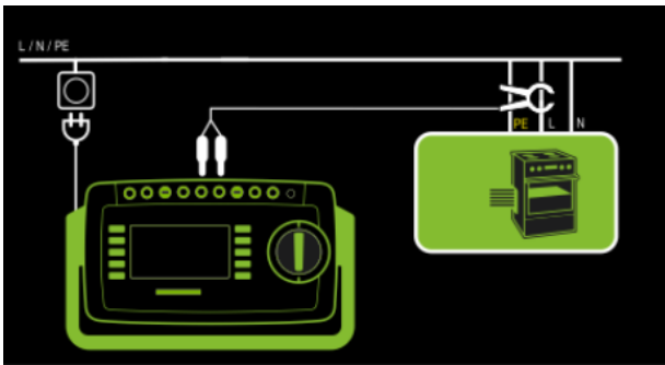
Abb. 150: Strom über Zange, Anschlussschaltbild
