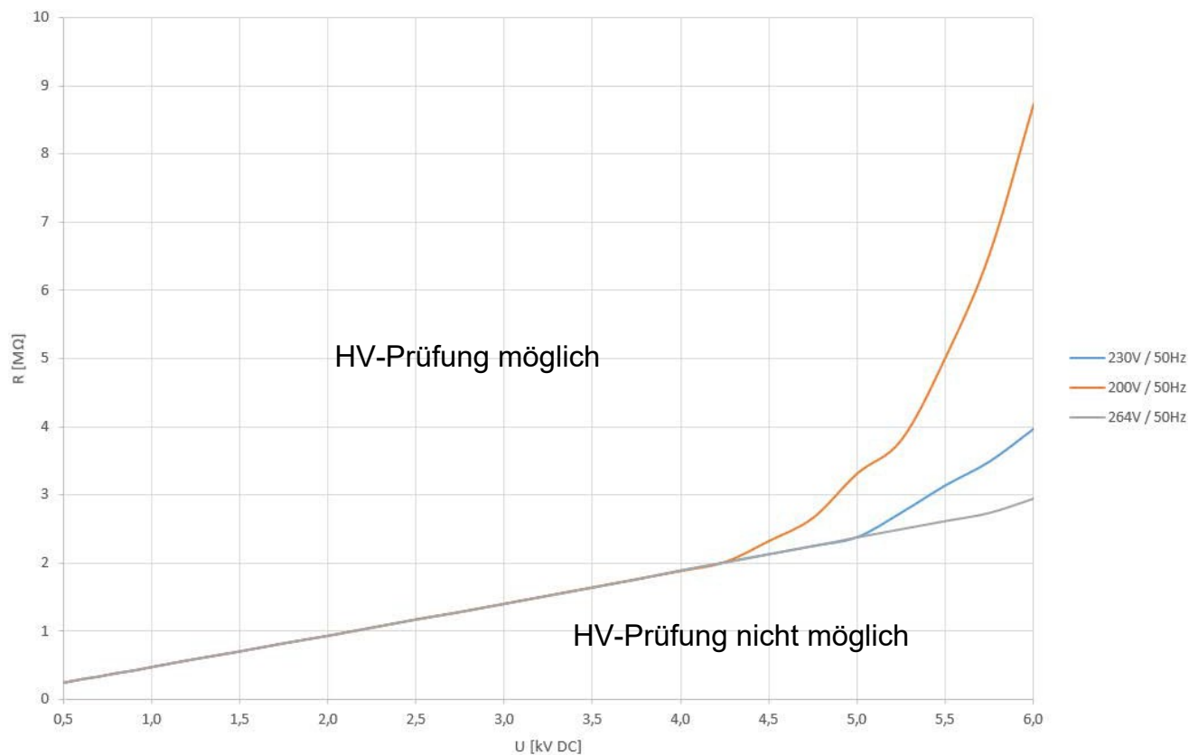
Abb. 3: Typische maximale Belastung der HV-Quelle in Abhängigkeit von der Versorgungsspannung bei 50 Hz
