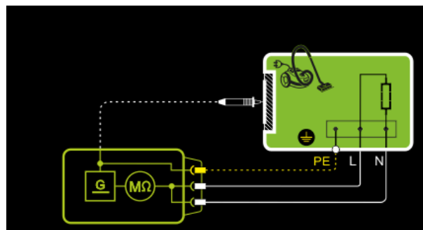
Abb. 56: Prüflinge der Schutzklasse II mit berührbaren elektrischen Teilen, Prinzipschaltbild
