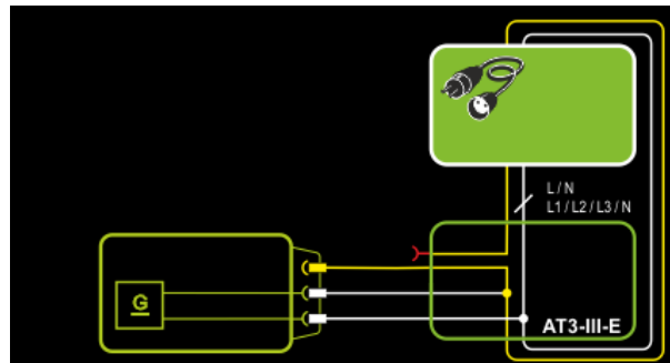
Abb. 145: Messung an 1- und 3-phasigen Verlängerungsleitungen mit AT3-I IIE, Prinzipschaltbild
