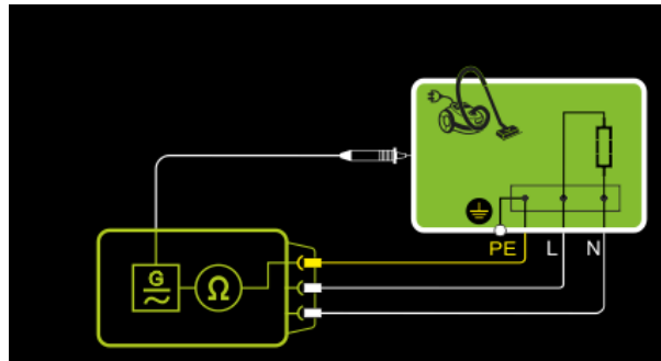
Abb. 41: Prüflinge der Schutzklasse I, Prinzipschaltbild
