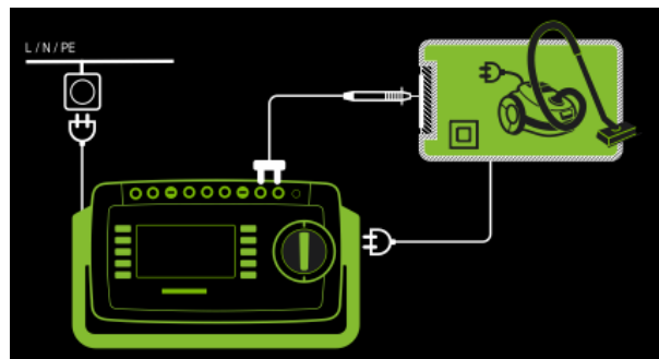
Abb. 95: Direktes Messverfahren, Anschlussschaltbild
