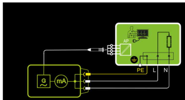
Abb. 118: Alternatives Messverfahren (Ersatz-Patientenableitstrom), Prinzipschaltbild
