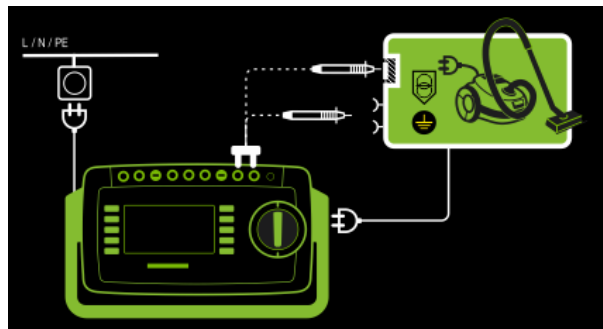
Abb. 61: Prüflinge der Schutzklasse I mit Ausgängen für Schutzkleinspannung, Anschlussschaltbild
