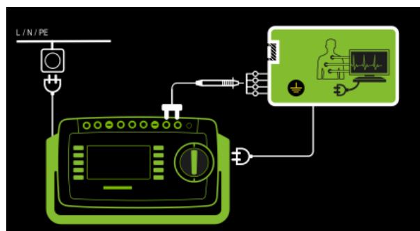
Abb. 117: Direktes Messverfahren, Anschlussschaltbild
