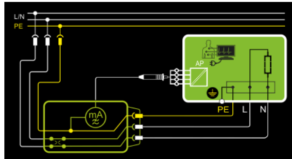
Abb. 123: Direktes Messverfahren, Prinzipschaltbild
