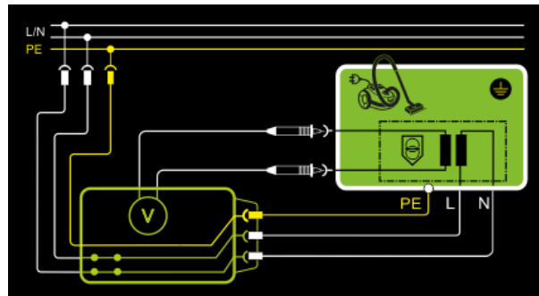
Abb. 133: Netz an Prüfdose, Prinzipschaltbild
