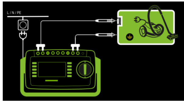
Abb. 103: Alternatives Messverfahren mit 2-Pol-Messung, Anschlussschaltbild
