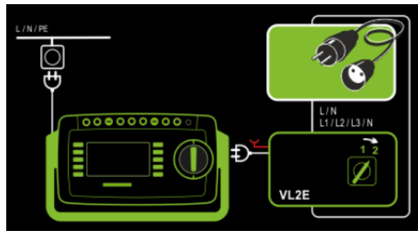
Abb. 144: Messung an 1- und 3-phasigen Verlängerungsleitungen mit VL2E, Anschlussbild
