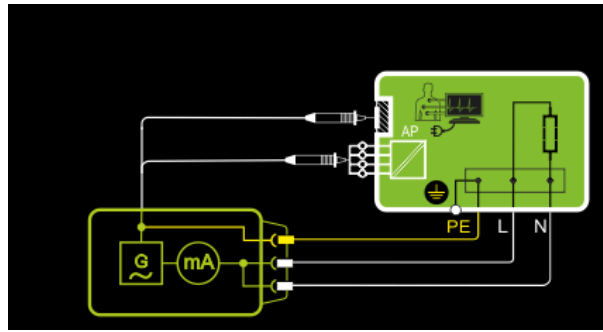
Abb. 109: Alternatives Messverfahren (Ersatz-Ableitstrom) Schutzklasse I, Prinzipschaltbild
