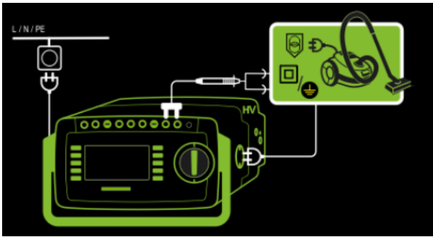
Abb. 78: Prüflinge der Schutzklasse II, Anschlussschaltbild
