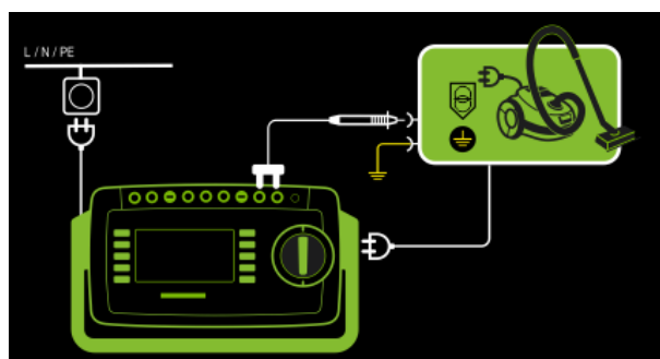
Abb. 129: Netz an Prüfdose, Anschlussschaltbild
