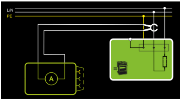
Abb. 149: Strom über Zange, Prinzipschaltbild
