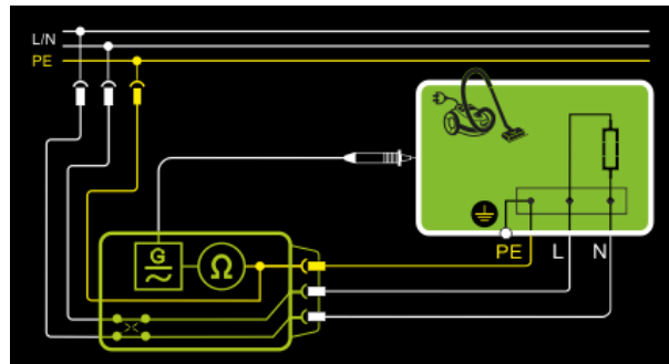
Abb. 45: Prüflinge der Schutzklasse I – Sonderfall Netzspannung an der Prüfdose (zur Prüfung von PRCDs), Prinzipschaltbild
