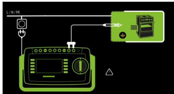
Abb. 131: Fest angeschlossener Prüfling, Anschlussschaltbild
