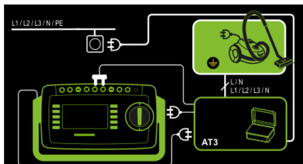
Abb. 90: Anschluss von 3-phasigen Prüflingen, Anschlussschaltbild
