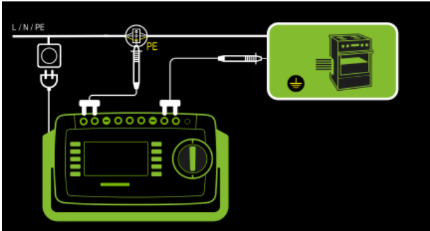
Abb. 52: 2-Pol-Messung an fest installierten Prüflingen, Anschlussschaltbild
