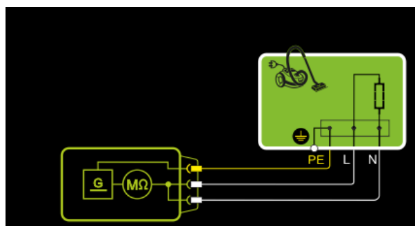
Abb. 54: Prüflinge der Schutzklasse I, Prinzipschaltbild
