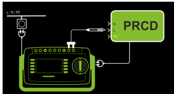
Abb. 138: Messung der Auslösezeit von Fehlerstrom-Schutzeinrichtungen, Anschlussschaltbild
