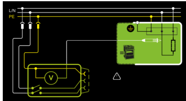
Abb. 130: Fest angeschlossener Prüfling, Prinzipschaltbild
