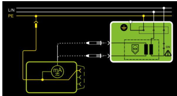
Abb. 100: Direktes Messverfahren bei fest installierten Prüflingen, Prinzipschaltbild
