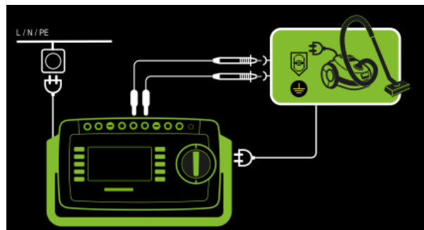
Abb. 134: Netz an Prüfdose, Anschlussschaltbild
