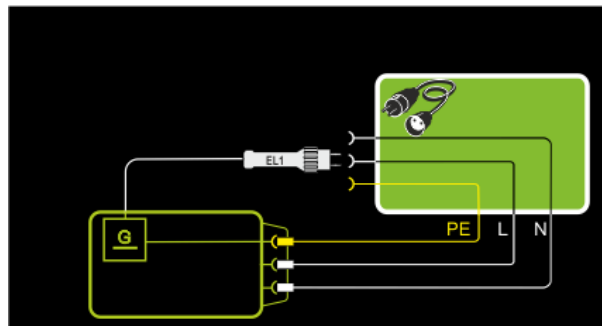
Abb. 43: Messung von R_{PE} an 1-phasigen Verlängerungsleitungen mit EL1, Prinzipschaltbild
