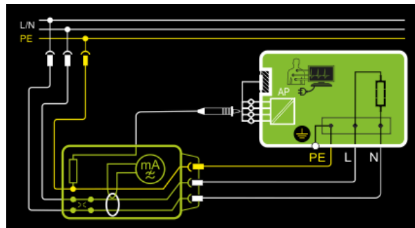
Abb. 106: Differenzstrommessverfahren Schutzklasse I, Prinzipschaltbild
