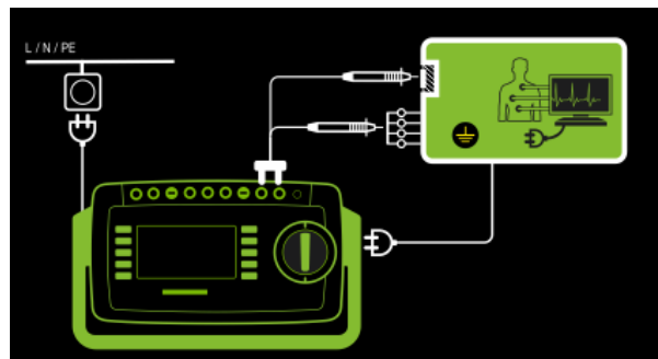
Abb. 108: Differenzstrommessverfahren Schutzklasse II, Anschlussschaltbild
