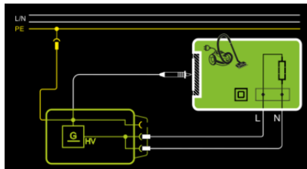
Abb. 75: Prüflinge der Schutzklasse II, Prinzipschaltbild
