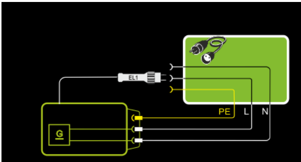
Abb. 141: Messung an 1-phasigen Verlängerungsleitungen mit EL1, Prinzipschaltbild
