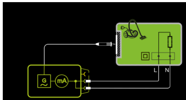
Abb. 98: Alternatives Messverfahren (Ersatz-Ableitstrom), Prinzipschaltbild
