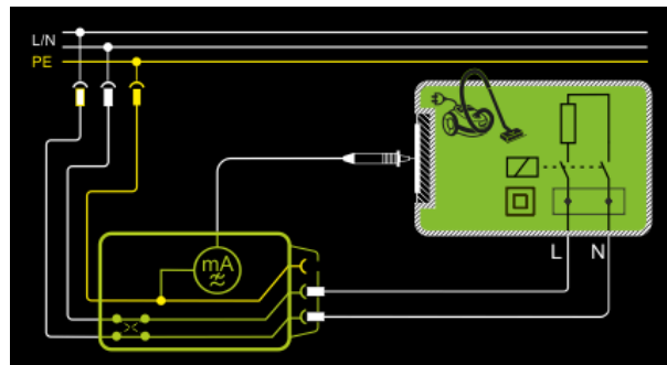
Abb. 94: Direktes Messverfahren, Prinzipschaltbild
