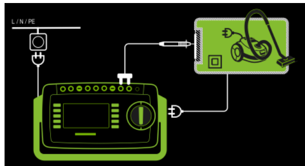
Abb. 97: Differenzstrommessverfahren, Anschlussschaltbild
