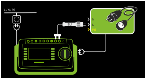
Abb. 142: Messung an 1-phasigen Verlängerungsleitungen mit EL1, Anschlussschaltbild
