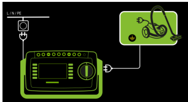
Abb. 88: Alternatives Messverfahren (Ersatz-Ableitstrom), Anschlussschaltbild
