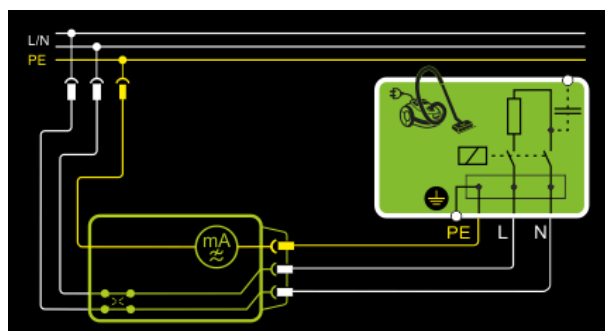
Abb. 83: Direktes Messverfahren, Prinzipschaltbild
