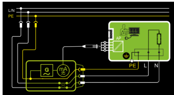
Abb. 116: Direktes Messverfahren, Prinzipschaltbild
