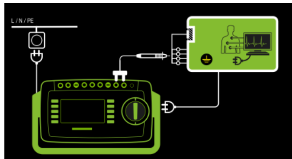
Abb. 107: Differenzstrommessverfahren Schutzklasse I, Anschlussschaltbild
