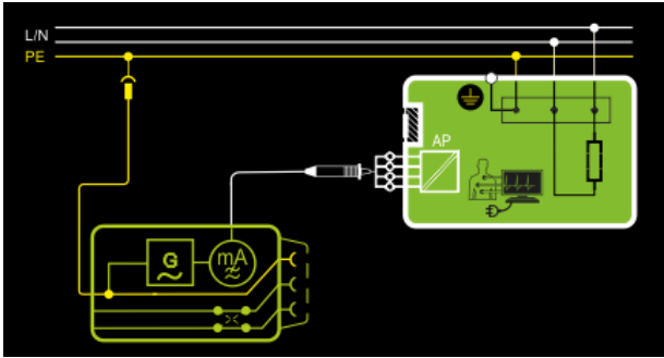
Abb. 120: Direktes Messverfahren, Prinzipschaltbild
