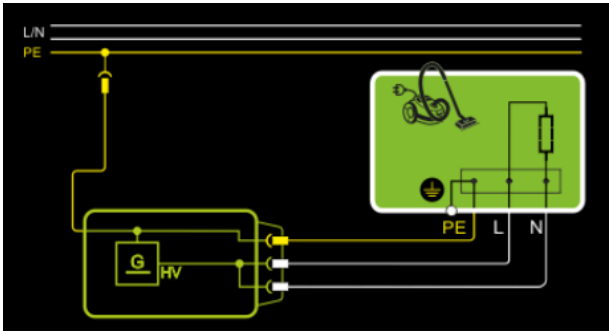
Abb. 73: Prüflinge der Schutzklasse I und Schutzklasse I+II, Prinzipschaltbild
