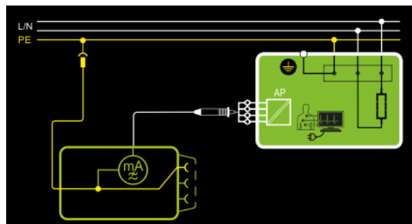
Abb. 125: Direktes Messverfahren, Prinzipschaltbild
