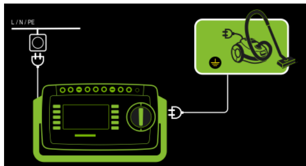
Abb. 140: Funktionstest, Anwendungsschaltbild
