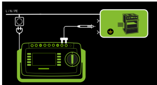
Abb. 101: Direktes Messverfahren bei fest installierten Prüflingen, Anschlussschaltbild
