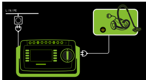
Abb. 84: Direktes Messverfahren, Anschlussschaltbild
