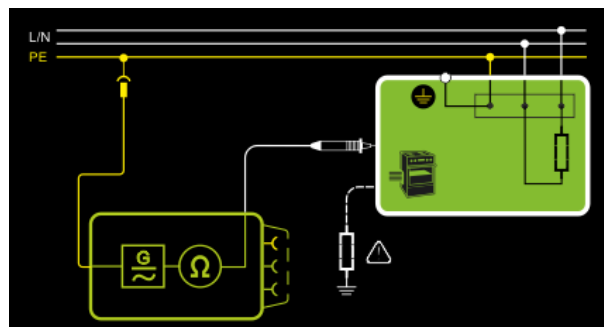
Abb. 47: Prüflinge der Schutzklasse I – fest installierte Prüflinge, Prinzipschaltbild
