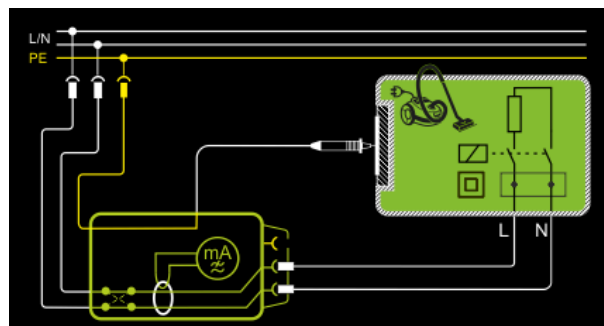
Abb. 96: Differenzstrommessverfahren, Prinzipschaltbild
