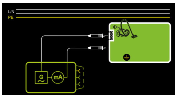
Abb. 102: Alternatives Messverfahren mit 2-Pol-Messung, Prinzipschaltbild
