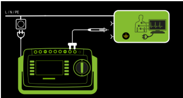
Abb. 126: Direktes Messverfahren, Anschlusschaltbild
