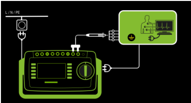
Abb. 119: Alternatives Messverfahren (Ersatz-Patientenableitstrom), Anschluss Schaltbild
