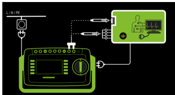
Abb. 105: Direktes Messverfahren, Anschlussschaltbild
