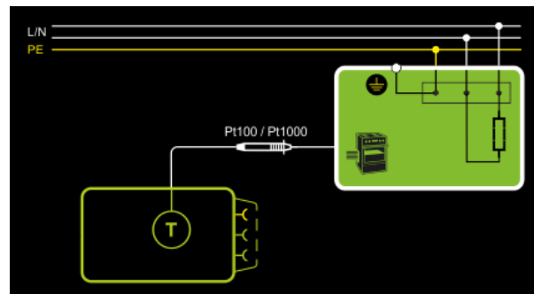
Abb. 147: Temperaturmessung, Prinzipschaltbild
