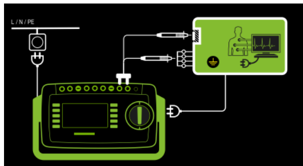
Abb. 110: Alternatives Messverfahren (Ersatz-Ableitstrom) Schutzklasse I, Anschlussschaltbild
