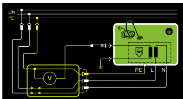
Abb. 128: Netz an Prüfdose, Prinzipschaltbild
