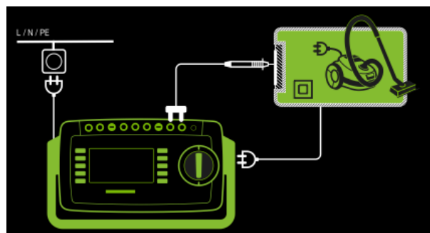
Abb. 99: Alternatives Messverfahren (Ersatz-Ableitstrom), Anschlussschaltbild
