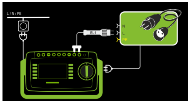
Abb. 44: Messung von R_{PE} an 1-phasigen Verlängerungsleitungen mit EL1, Anschlussschaltbild
