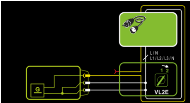
Abb. 143: Messung an 1- und 3-phasigen Verlängerungsleitungen mit VL2E, Prinzipschaltbild
