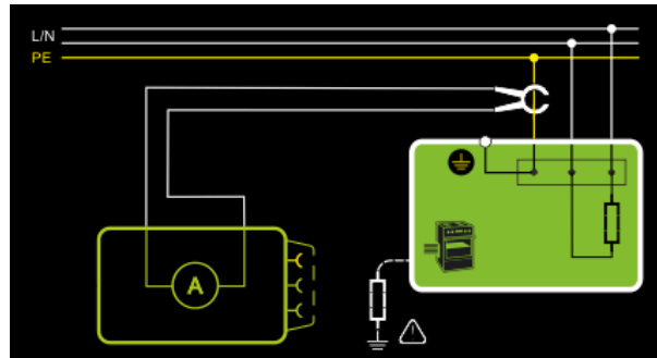
Abb. 91: Messung des Schutzleiterstroms über Zangenstromsensor mit Spannungsausgang bei fest installierten Prüflingen, Prinzipschaltbild
