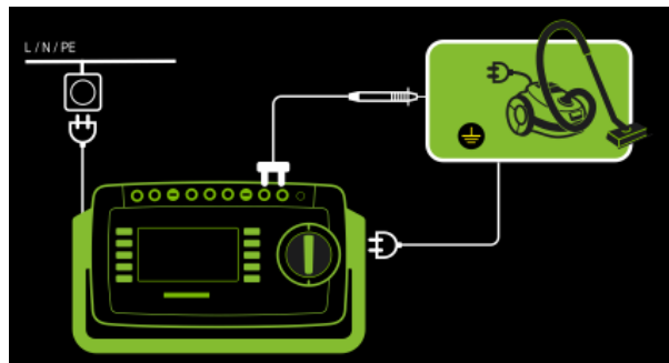
Abb. 42: Prüflinge der Schutzklasse I, Anschlussschaltbild
