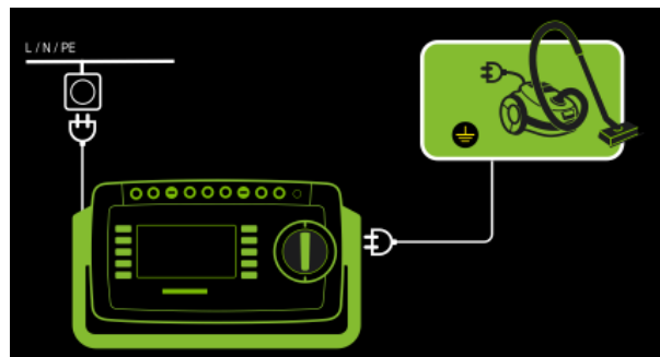
Abb. 86: Differenzstrommessverfahren, Anschlussschaltbild
