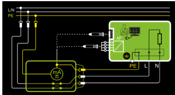
Abb. 104: Direktes Messverfahren, Prinzipschaltbild
