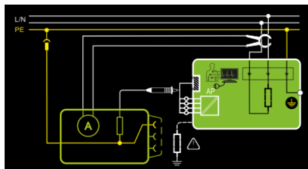
Abb. 113: Messverfahren mit Zangenstromsensor bei fest installierten Prüflingen, Prinzipschaltbild
