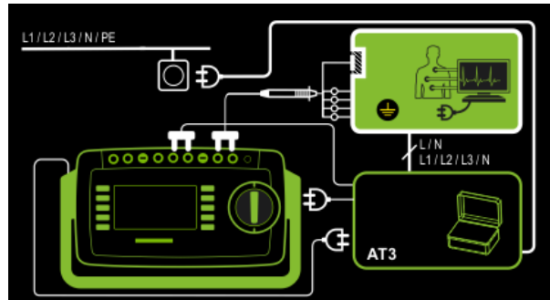
Abb. 112: Differenzstrommessverfahren, Anschlussschaltbild
