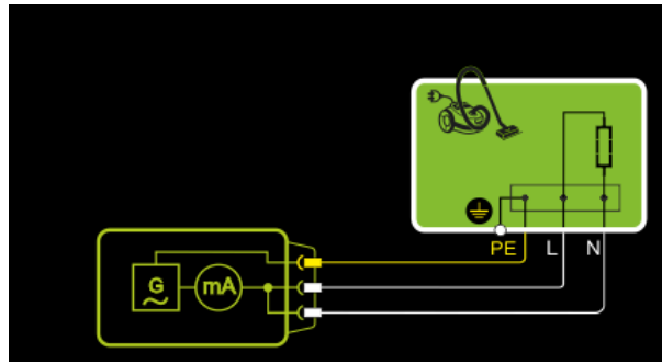
Abb. 87: Alternatives Messverfahren (Ersatz-Ableitstrom), Prinzipschaltbild
