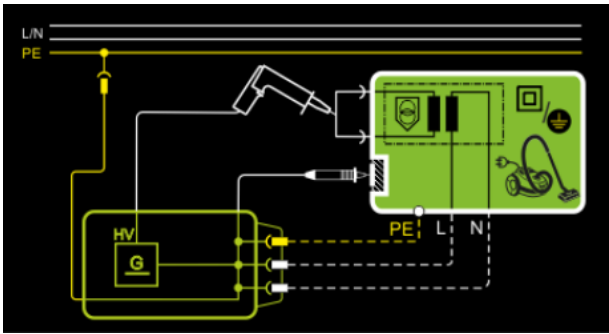
Abb. 79: Sonstige oder beliebige Prüflinge, Prinzipschaltbild
