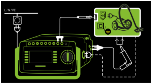
Abb. 80: Sonstige oder beliebige Prüflinge, Anschlussschaltbild
