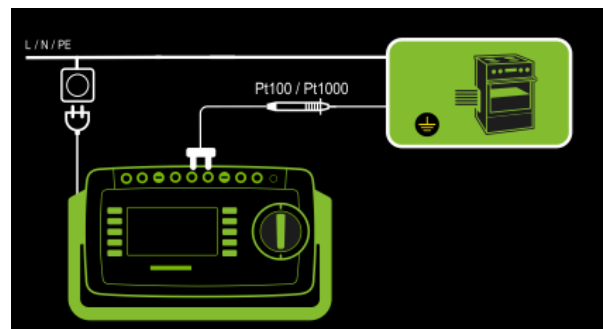
Abb. 148: Temperaturmessung, Anschlussschaltbild
