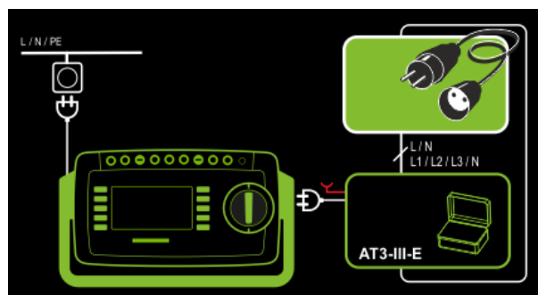
Abb. 146: Messung an 1- und 3-phasigen Verlängerungsleitungen mit AT3-I IIE, Anschlussbild
