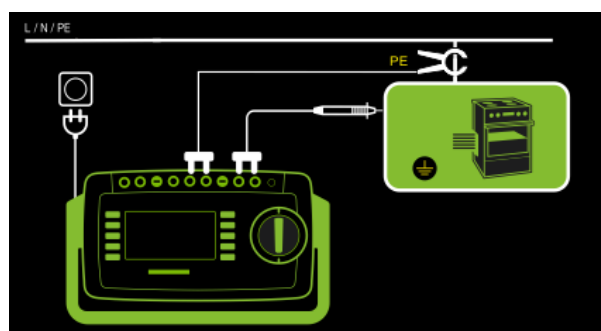
Abb. 50: Messung über Zangenstromsensor an fest installierten Prüflingen, Anschlussschaltbild
