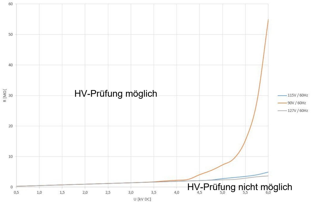
Abb. 4: Typische maximale Belastung der HV-Quelle in Abhängigkeit von der Versorgungsspannung bei 60 Hz
