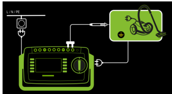
Abb. 46: Prüflinge der Schutzklasse I – Sonderfall Netzspannung an der Prüfdose (zur Prüfung von PRCDs), Anschlussschaltbild
