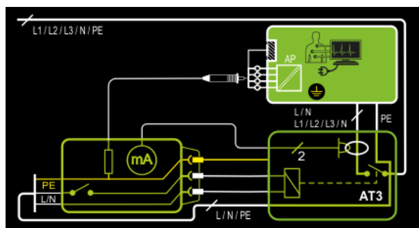
Abb. 111: Differenzstrommessverfahren, Prinzipschaltbild
