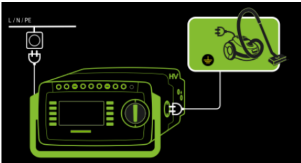
Abb. 74: Prüflinge der Schutzklasse I und Schutzklasse I+II, Anschlussschaltbild
