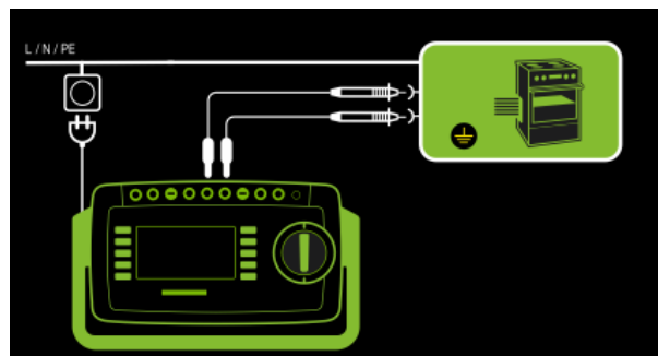
Abb. 136: Fest angeschlossener Prüfling, Anschlussschaltbild
