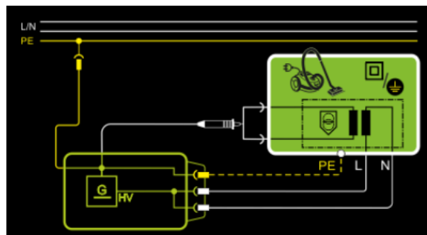
Abb. 76: Prüflinge der Schutzklasse II, Prinzipschaltbild
