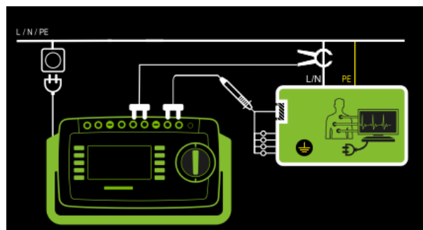
Abb. 114: Messverfahren mit Zangenstromsensor bei fest installierten Prüflingen, Anschlussschaltbild
