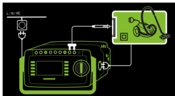
Abb. 77: Prüflinge der Schutzklasse II, Anschlussschaltbild
