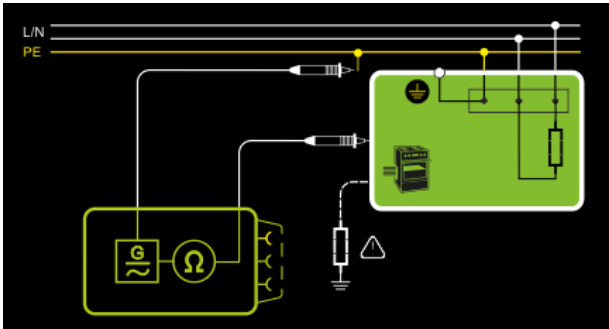
Abb. 51: 2-Pol-Messung an fest installierten Prüflingen, Prinzipschaltbild
