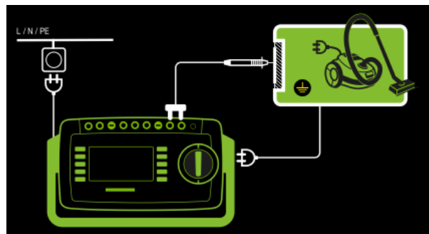
Abb. 71: Prüflinge der Schutzklasse I mit berührbaren elektrischen Teilen, Anschlussschaltbild
